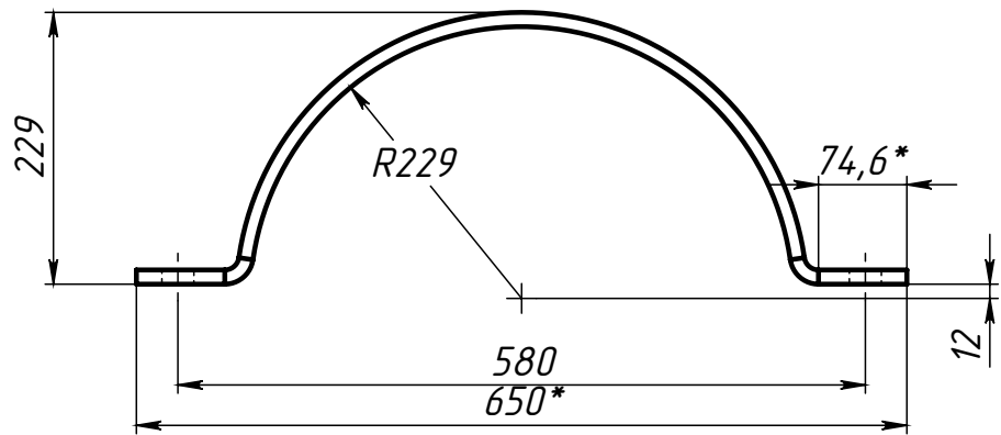
Поз.4 (Полухомут)
