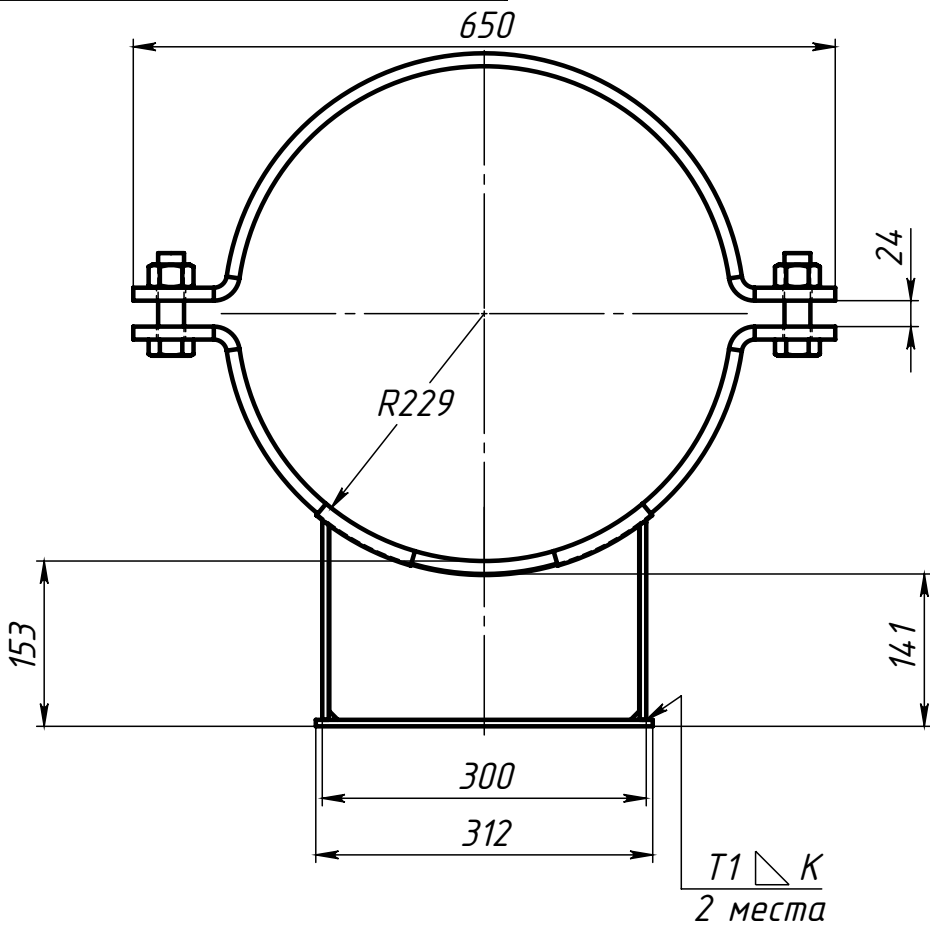
Поз.4 (Полухомут)
